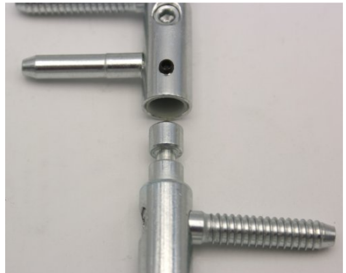
Detail zabezpečení proti bočnímu pohybu:
